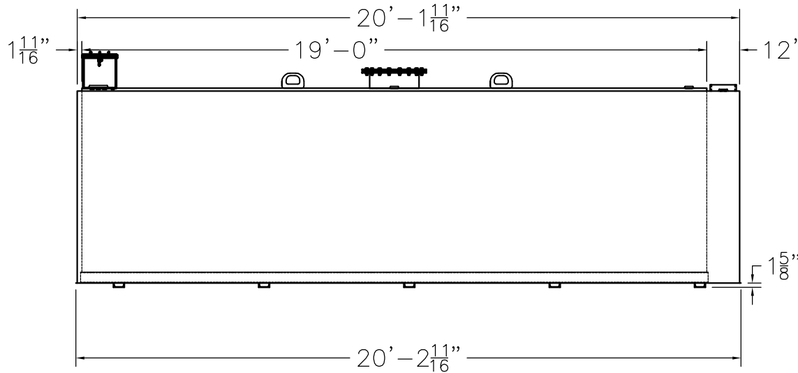
ELEVATION
